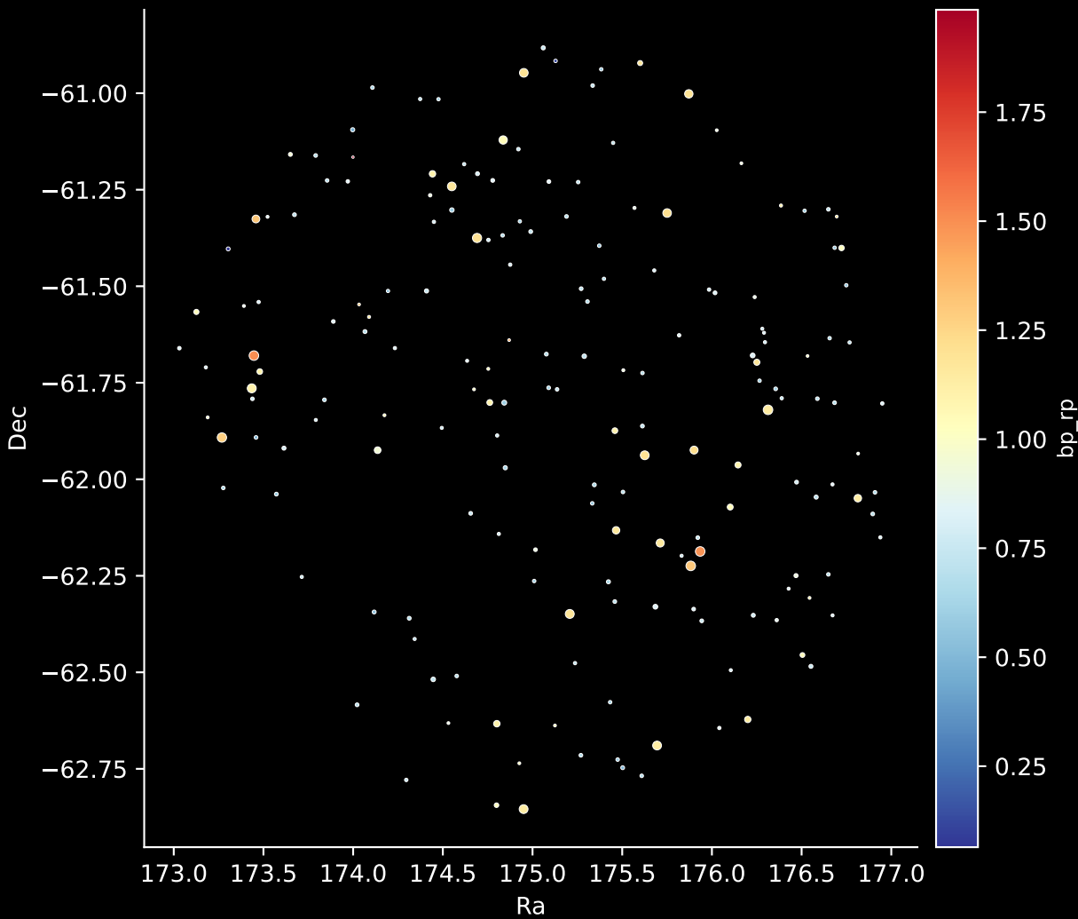
GALAH DR4 Field: [7156] Stars: 182
